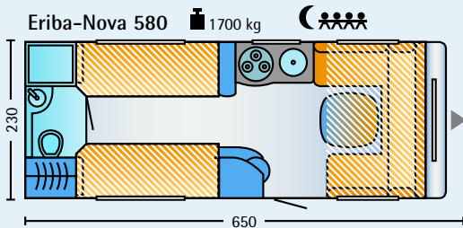
Längs-Einzelbetten / Rundsitzgruppe
