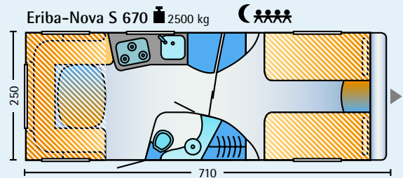
Rundsitzgruppe / Längs-Einzelbetten
