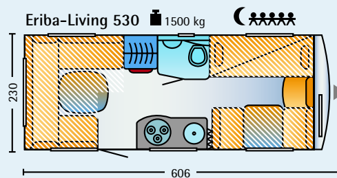
Rundsitzgruppe / Kinderzimmer-Variante
