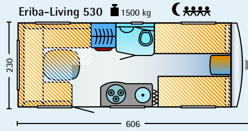
Rundsitzgruppe / Längs-Einzelbetten
