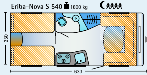
Längs-Einzelbetten / Rundsitzgruppe
