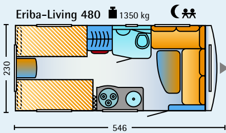
Längs-Einzelbetten / L-Sitzgruppe
